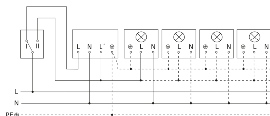
Diagrama electrónico conexión del acoplador pulsador de 4 vías al APC DALI2
